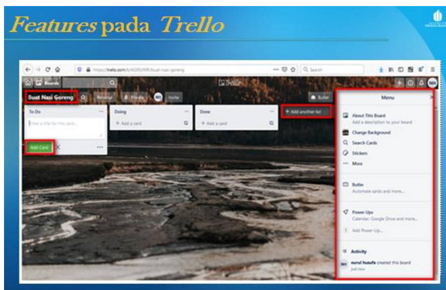
Gambar 1. Features-features yang terdapat pada Trello
